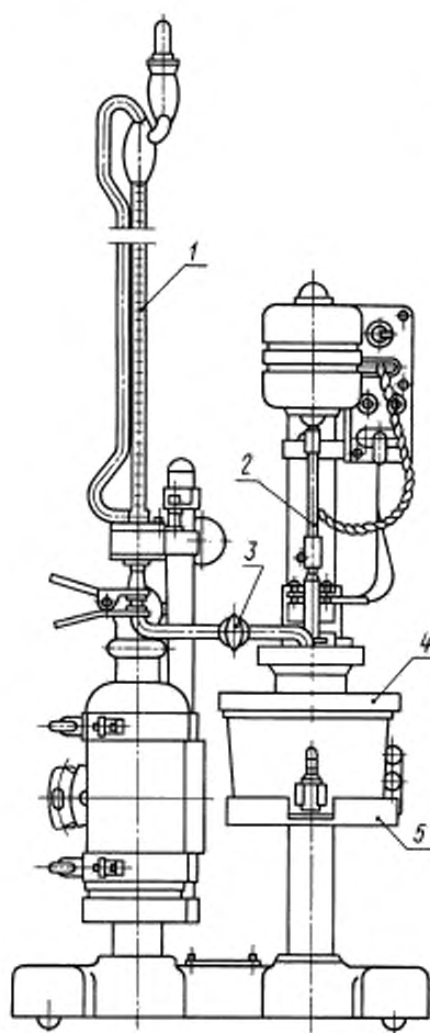
1 — бюретка; 2 — мешалка; 3 — кран бюретки; 4 — сосуд для охлаждения; 5 — столик титровального стенда
