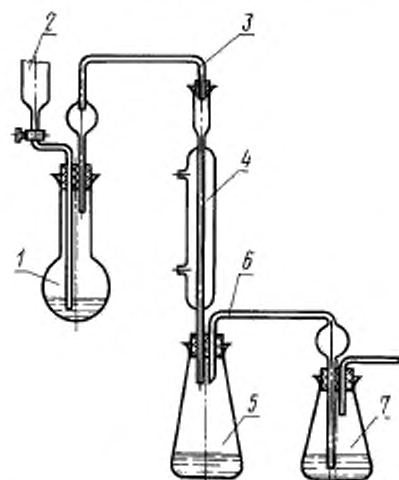
1 — перегонная колба вместимостью 500 см 3 ; 2 — капельная воронка; 3 — насадка с брызгоуловителем; 4 — водяной холодильник; 5 — приемник (коническая колба вместимостью 250 см 3 ); 6 — стеклянная трубка с грушевидным расширением; 7 — контрольный приемник (коническая колба вместимостью 250 см 3 )
