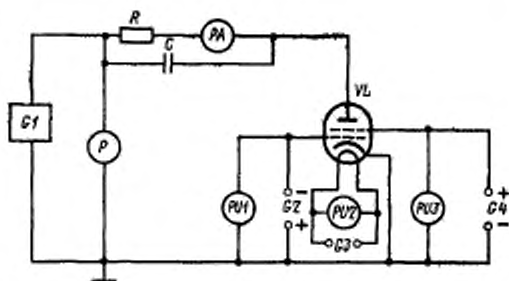
С — конденсатор; G1 — генератор импульсов; G2, G4 — источники постоянного тока; G3 — источник переменного или переменного тока; PA — микроамперметр постоянного тока; P — устройство для измерения импульсного напряжения; PU1, PU3 — вольтметры постоянного тока; PU2 — вольтметр постоянного или переменного тока; R — резистор; VL — испытуемая лампа
