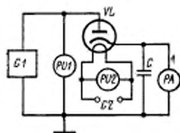
C —конденсатор; G1 —генератор синусоидального напряжения; G2 —источник постоянного или переменного тока; PA —миллиамперметр постоянного тока; PU1 —вольтметр переменного тока; PU2 —вольтметр постоянного или переменного тока; VL —испытуемая лампа
