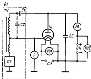
G1 — генератор импульсного напряжения ( C1 , C2 — конденсаторы; TV — импульсный трансформатор; G2 — генератор тока); C3 — конденсатор; G3 — источник постоянного или переменного тока; G4 — источник постоянного тока; PA — миллиамперметр постоянного тока; PU1 — вольтметр постоянного или переменного тока; PU2 — вольтметр постоянного тока; P — измерительное устройство; VL — испытуемая лампа
