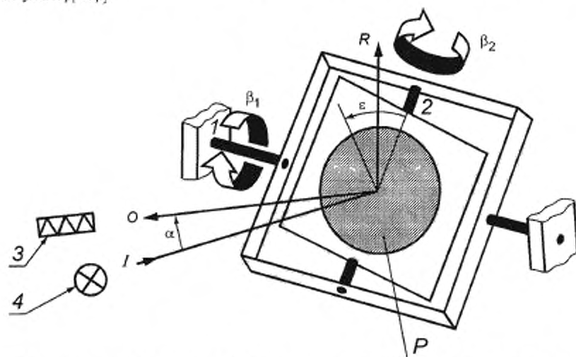
Рисунок 2 — Гониометрический механизм и система углов МКО
