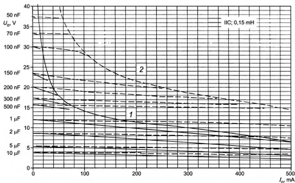
Рисунок С.7а — Диаграмма для 0,15 мГн (продолжение)
