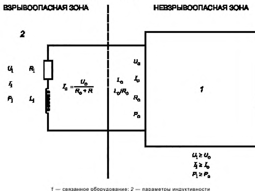
Рисунок D.1 — Типовая индуктивная цепь
