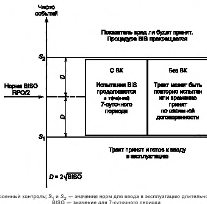
Рисунок 4.14 — Схема процедуры принятия решения о вводе в эксплуатацию
