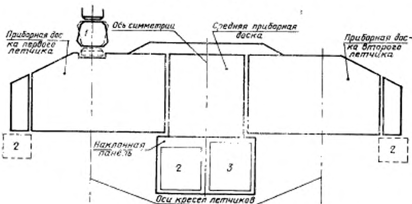
Размещение пилотажно-навигационных индикаторов вне приборной доски и в ее вырезах
