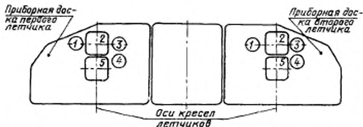
Размещение группы основных пилотажно-навигационных индикаторов на приборных досках первого и второго летчиков
