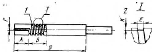
1—вытяжная канавка; 2—канавка в увеличенном виде
