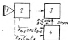
1 — испытательная таблица; 2 — камерный канал; 3 — ВКУ по п. 2.1.6; 4 — измеритель совмещения растров по п. 2.1.10
