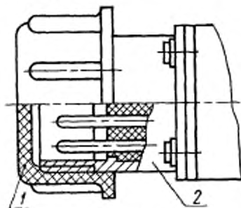
1 — крышка 1-М27×1,5—1П; 2 — соединитель
