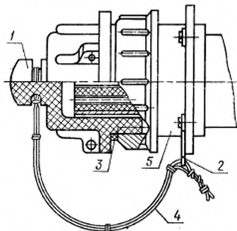
1 — крышка 2-M24×1—3Д; 2 — ушко 3.4; 3 — прокладка 31, марка резины; 4 — леска 0,6 мм l=300 мм; 5 — соединитель.
