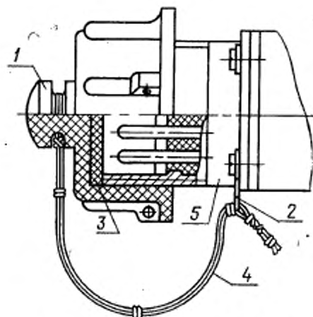
1 — крышка 1-M24×1; 2 — ушко 3.4; 3 — прокладка 10, марка резины; 4 — капроновая нить ЗК; l=300 мм; 5 — соединитель.
