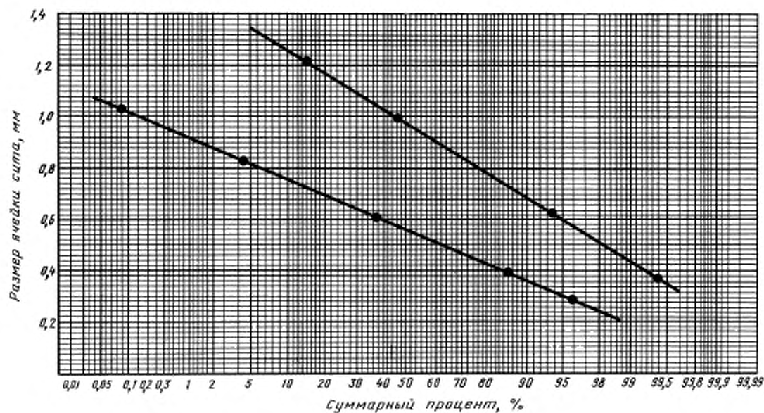
ГРАФИК ЗАВИСИМОСТИ СУММАРНОГО ПРОЦЕНТА ИОНИТА ОТ РАЗМЕРА ЯЧЕЙКИ СИТА
