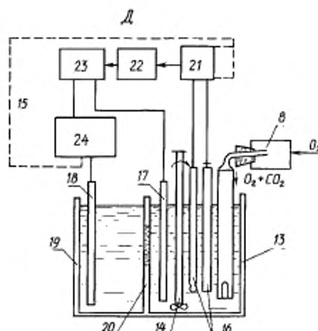
Схема экспресс-газоанализатора
