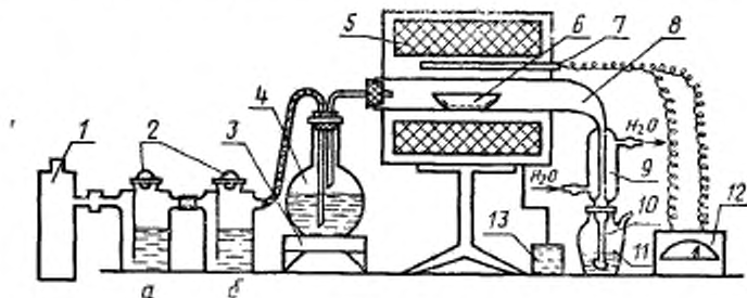
1 — баллон с газом; 2 — склянки для промывания газов (а — с концентрированной серной кислотой; б — с дистиллированной водой); 3 — электрод; 4 — парообразователь; 5 — трубчатая электроды сопротивления; 6 — лодочка фарфоровая; 7 — платино-платинородиевая термопара; 8 — кварцевая трубка; 9 — холодильник; 10 — отводная трубка; 11 — колба-приемник; 12 — милливольтметр; 13 — трансформатор напряжения для регулирования температуры печи
