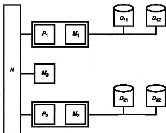
Рисунок А.8 — Структурная схема мультипроцессора
