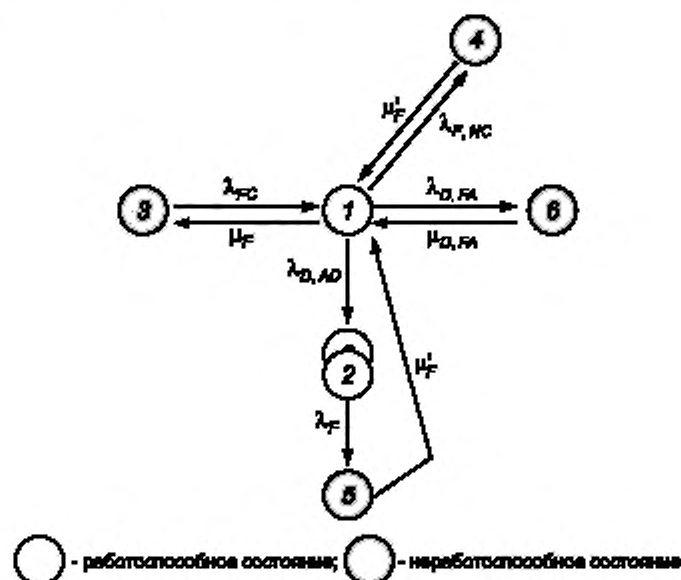
Рисунок А.7 — Диаграмма состояний и переходов
