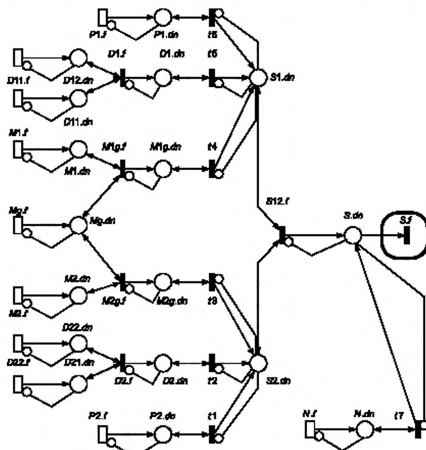
Рисунок А.9 — Сеть Петри мультипроцессорной системы
