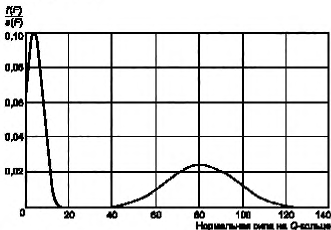
Рисунок А.12 — Пример применения критерия прочности напряжений
