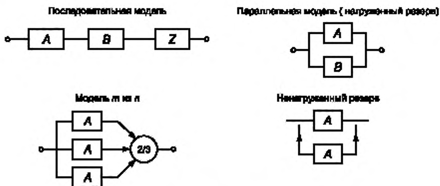
Рисунок A.5 — RBD для независимых блоков
