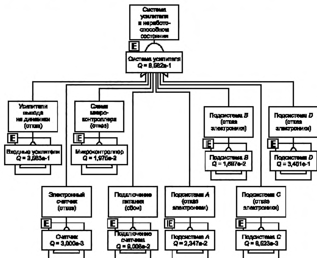
Рисунок A.2 — Дерево неисправностей для аудиоусилителя
