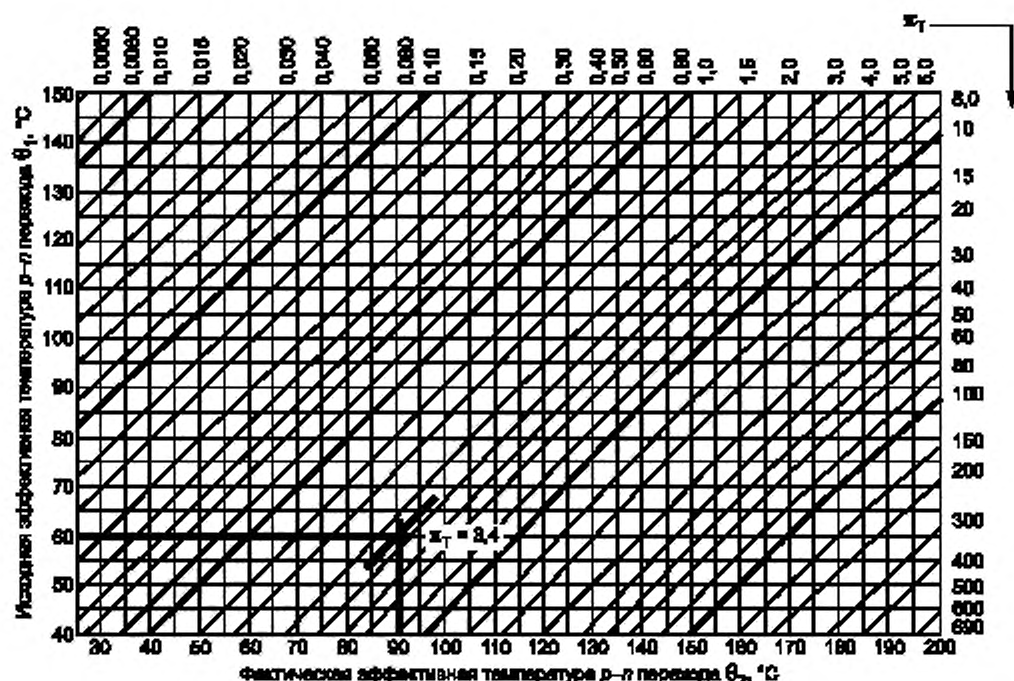
Рисунок A.1 — Зависимость интенсивности отказов от температуры
