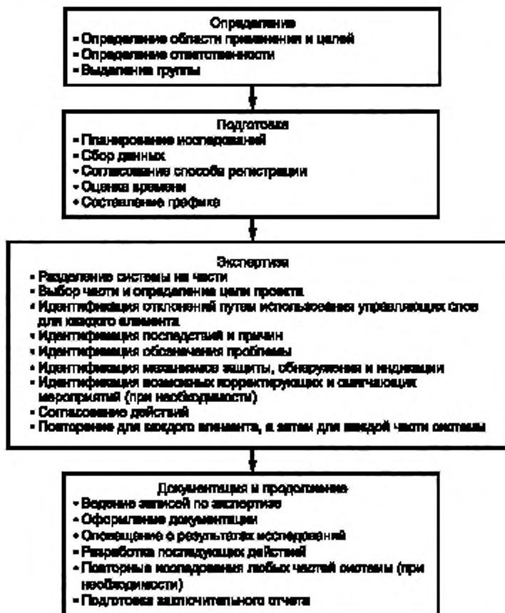
Рисунок А.10 — Этапы исследования HAZOP
