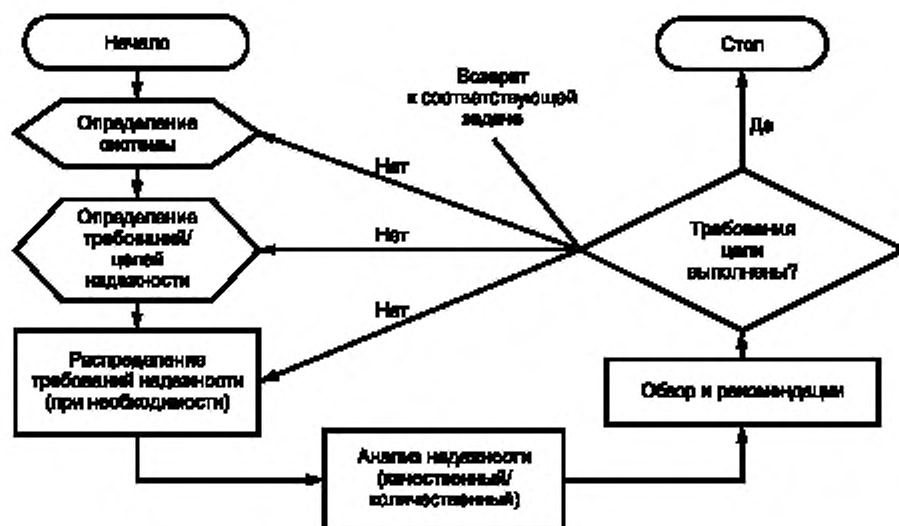
Рисунок 1 — Общая процедура анализа надежности
