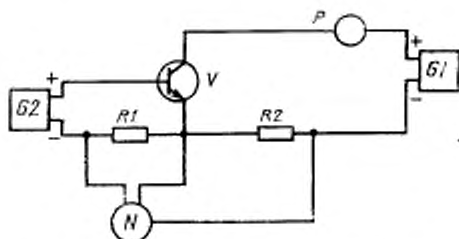
R1, R2 — безиндуктивные измерительные резисторы с малым сопротивлением; N — осциллоскоп; P — измеритель амплитудных значений тока; G1 — источник напряжения; G2 — источник тока; V — испытуемый транзистор
