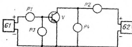
P1 , P2 — измерители амплитудных значений тока; P3 , P4 — измерители мгновенных значений напряжения; G1 — источник тока; G2 — источник напряжения; V — испытательный транзистор
