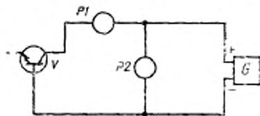
P1 — измеритель мгновенных значений тока; P2 — измеритель амплитудных значений напряжения; G — источник напряжения; V — испытываемый транзистор
