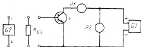
G1, G2 — источники напряжения; P1 — измеритель мгновенных значений тока; P2 — измеритель амплитудных значений напряжения; R_{БЭ} — резистор в цепи базы; V — испытываемый транзистор
