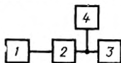
1—ЭП (ЭПУ) с грампластинкой (п. 4.2.14); 2—прибор (п. 4.2.2); 3—анализатор спектра (п. 4.2.3); 4—вольтметр (п. 4.2.7)
