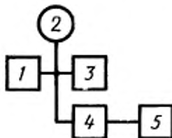
1—ЭФ с грампластинкой (пп. 4.2.16 и 4.2.12); 2—вольтметр (п. 4.2.7); 3—эквивалент нагрузки (п. 4.2.22); 4—прибор (п. 4.2.2); 5—регистратор уровня (п. 4.2.9)
