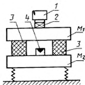
1—вибратор; 2—датчик силы; 3—испытуемые виброизоляторы; 4—датчик виброускорения; M_1 — грузоподъемная масса; M_2 —испы- тательная масса
