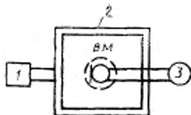
1 — низкочастотный генератор сигналов (п. 1.2.1); 2 — устройство для испытаний микрофонов на воздействие электромагнитного поля (п. 1.2.3); 3 — анализатор спектра (п. 1.5) или селективный вольтметр (п. 1.6); ВМ — испытуемый микрофон
