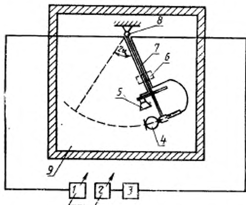
1 — низкочастотный генератор сигналов (п. 1.2.1); 2 — анализатор спектра (п. 1.5); 3 — самописец уровня (п. 1.2); 4 — испытуемый микрофон; 5 — излучатель (п. 1.11.2); 6 — инерционная масса; 7 — кронштейн; 8 — горизонтальная ось; 9 — звукомерная заглушенная камера (п. 1.18)
