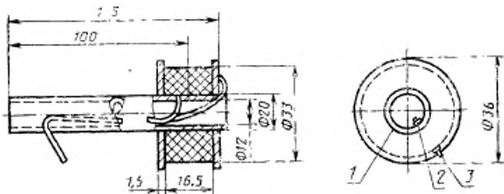
4500 витков эмалированного медного провода диаметром 0,13 мм; R=500\ \text{Ом} ; 1 — изоляционный материал; 2 — вывод первого витка, 3 — вывод последнего витка
