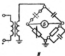
Схема с заземленной диагональю
