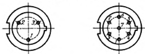
Схема расположения контактов вилки (вид со стороны пайки проводов)
