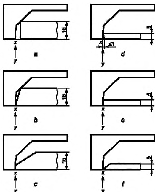
Случаи а) и б) — несоответствие; случаи в), г), д), е), ф) — соответствие, но подтвержденное испытаниями по 11.102.8 с использованием калибра
