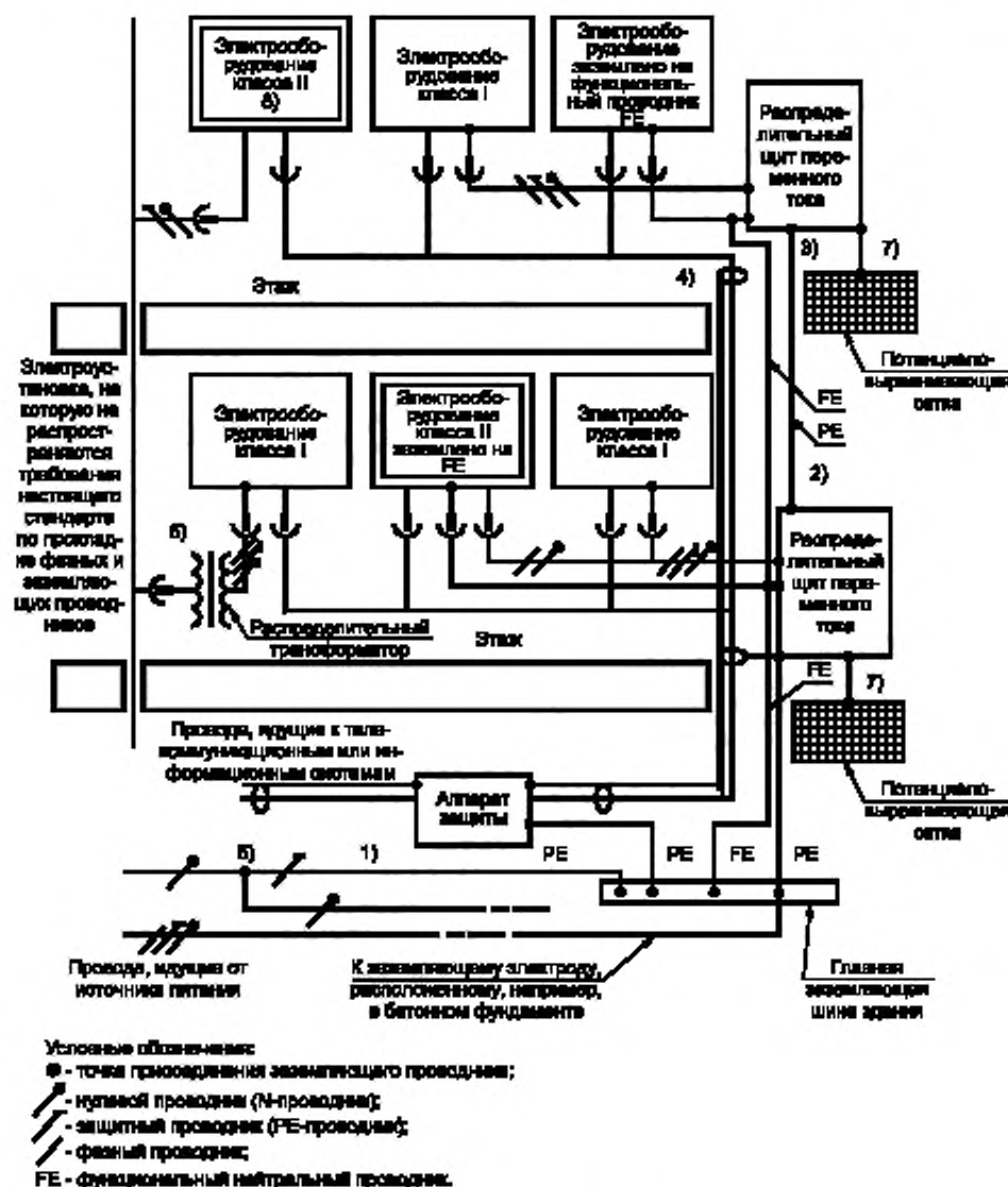
1) — PE-проводник; 2) — распределительный щит; 3) — уравнивание электрических потенциалов; 4) — экранированный провод; 5) — нулевой провод; 6) — разделительный трансформатор; 7) — локальное УЗЭП; 8) — электрооборудование
