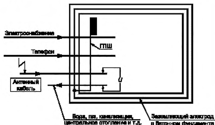
Рисунок 3а — Односторонний ввод (предпочтителен, U = 0 )
