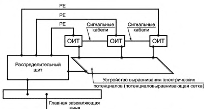
Рисунок В.2 — Локальное устройство выравнивания электрических потенциалов
