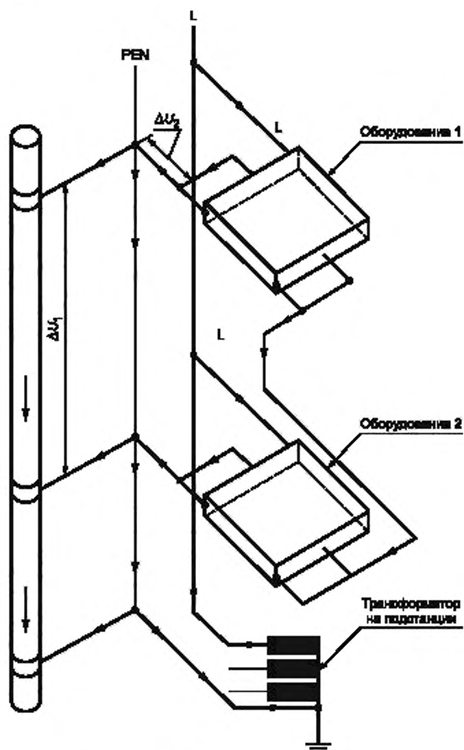
Рисунок 2а — Система заземлення типу TN-C
