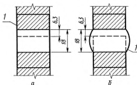
1 — образец ткани с покрытием; а — открытое положение; б — провисание образца
