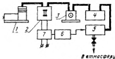
Блок-схемы приборов для измерения массовой доли газов:
