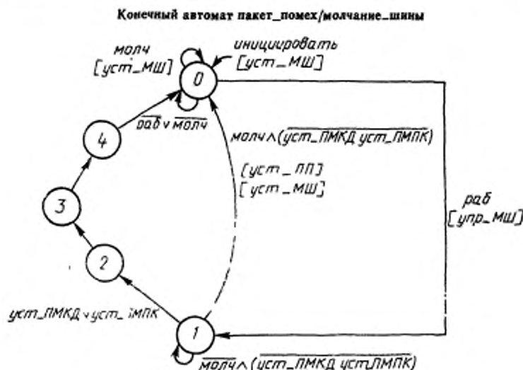
Черт. 5.8
