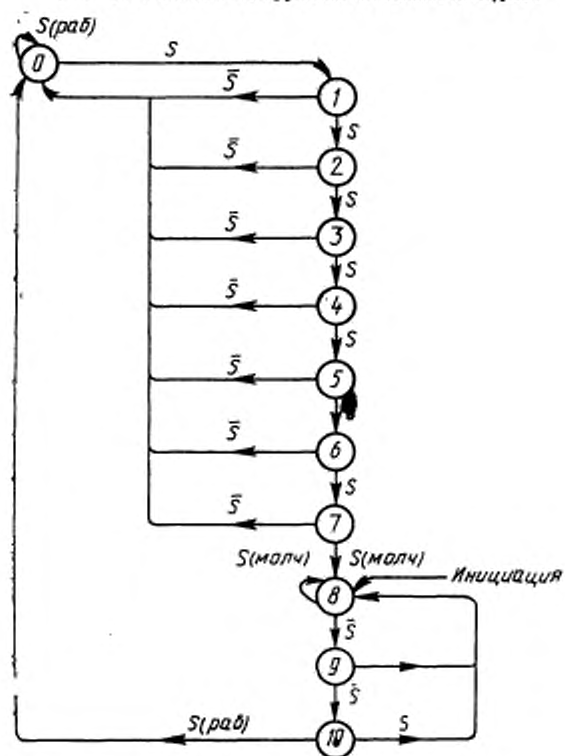
Конечный автомат «Обнаружение состояния молч/раб»
