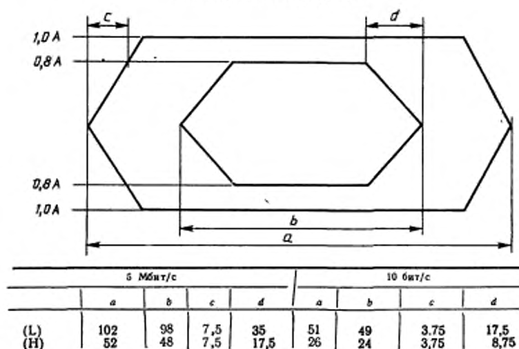
«Глазообразная» конфигурация
