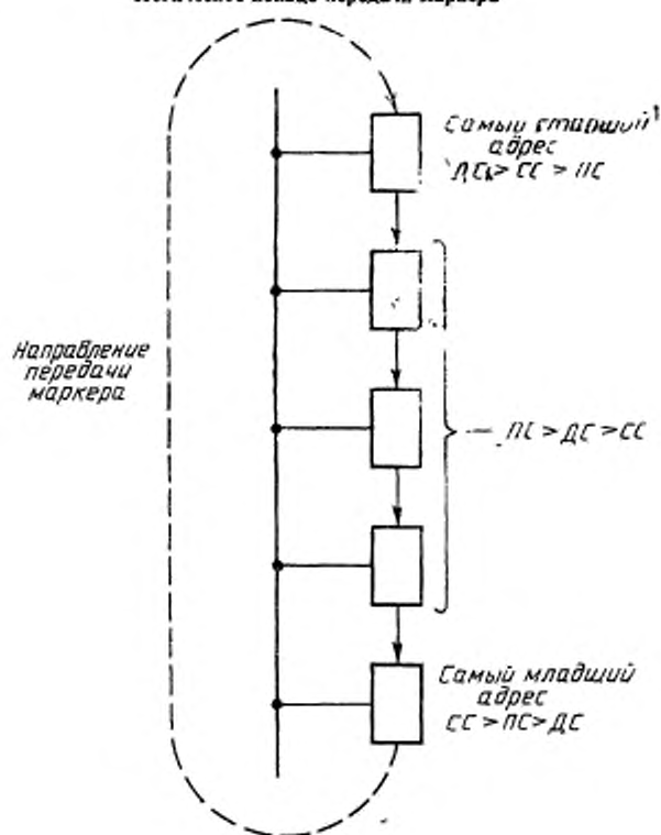
Черт. 6.2
