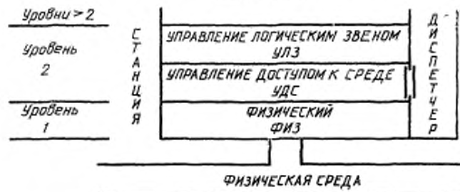
Черт. 3.1
