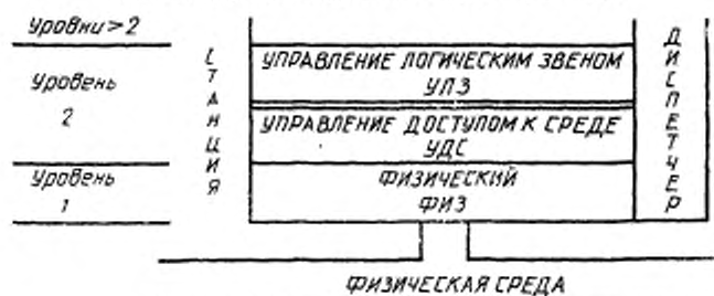
Черт. 2.1
