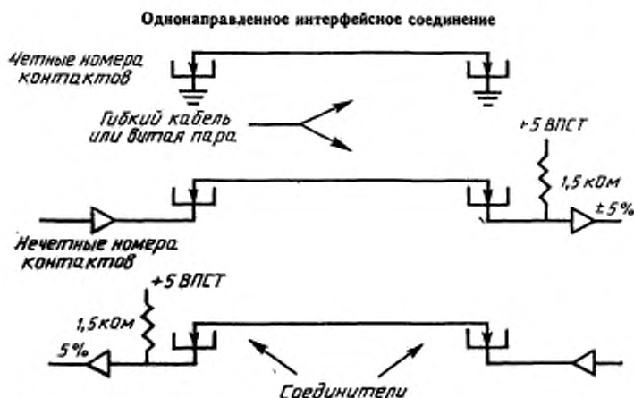
Черт. 10.2
