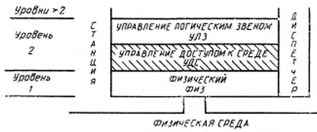
Черт. 5.1
