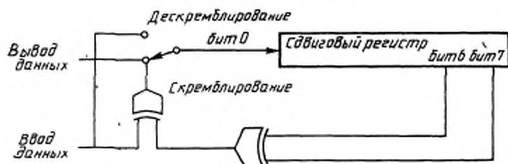
Черт. П7.2
