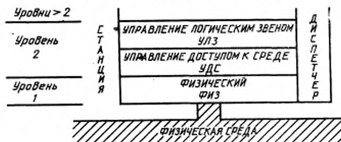
Черт. 17.1
