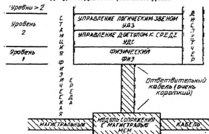
Черт. 19.2
