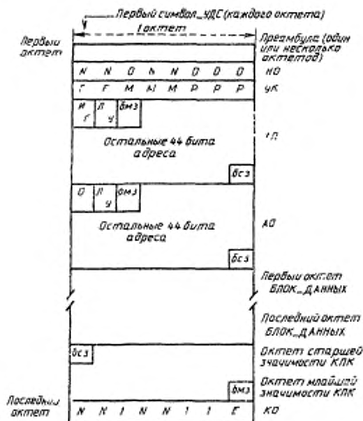
Черт. 6.1
