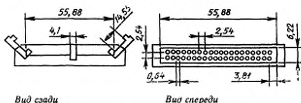
Розетка одинарного интерфейсного соединителя
