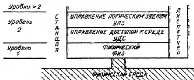
Черт. 19.1
