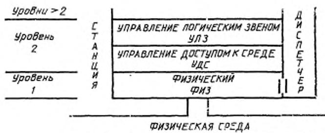
Черт. 9.1
