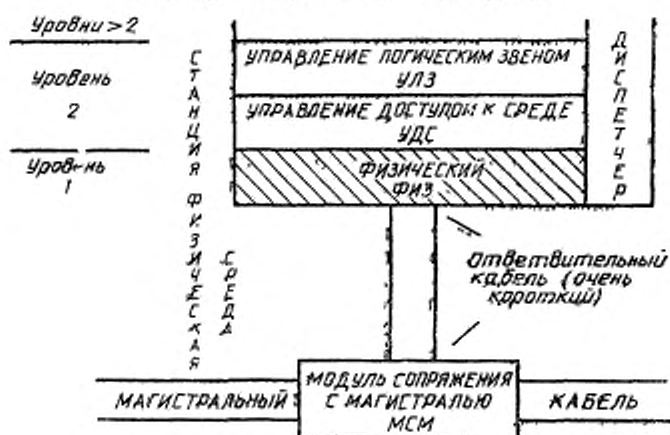
Черт. 18.2
