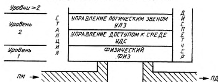
Черт. 17.2
