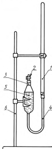
1 — бюретка; 2 — кран; 3 — пробка; 4 — резиновая трубка; 5 — резервуар; 6 — штатив
