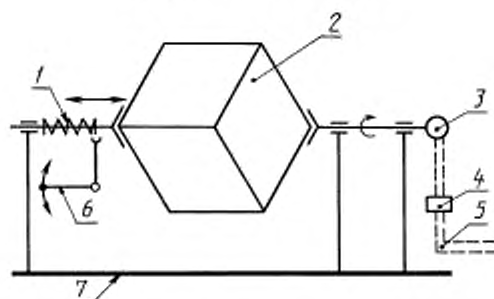
1 — пружина; 2 — куб; 3 — микрометр; 4 — реле времени; 5 — подача энергии; 6 — рычаг; 7 — станция
