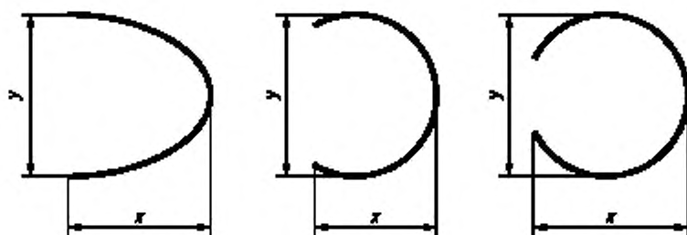
Рисунок 2 — Размеры манжеты
