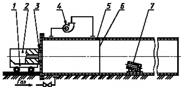
1 — тележка; 2 — канальная мортра; 3 — люк штреха; 4 — вентилятор для перемешивания метановоздушной смеси; 5 — труба штреха; 6 — диафрагма; 7 — мортра для распыления угольной пыли
