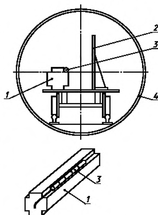
1 — уголовая мортра; 2 — отражательная стенка; 3 — испытуемый заряд ВВ; 4 — штрэк
