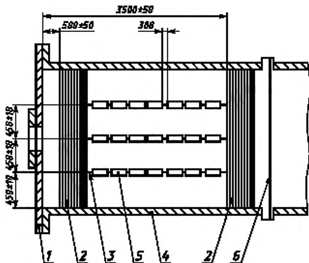
1 — дно трубы штрека; 2 — деревянная рудничная стойка; 3 — капроновая леска или провод; 4 — стенка трубы штрека; 5 — испытуемый заряд ВВ; 6 — диафрагма или шторный затвор
