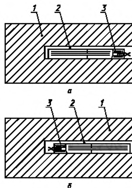
a — прямое инициирование; б — обратное инициирование 1 — канальная мортра; 2 — несеквойный канал, 3 — заряд ВВ с электродетонатором
