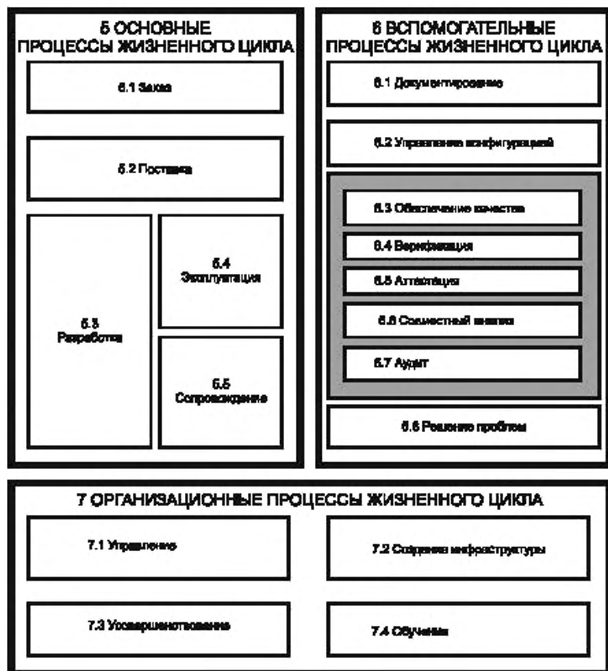
Рисунок 1 — Структура стандарта
