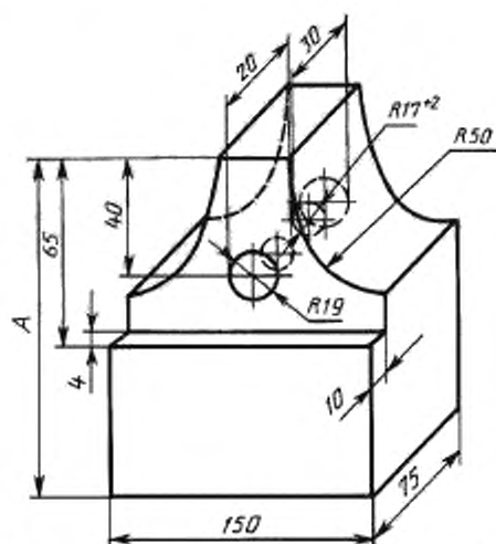
Рисунок 1 — Сводовые изделия номеров 1, 2
