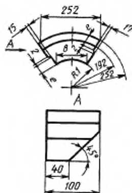
Рисунок 26 — Секторные изделия номеров 67, 69
