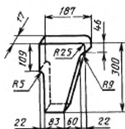
Рисунок 5 — Сводное изделие номер 6
