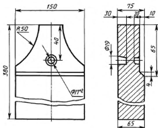
Рисунок 2 — Сводовое изделие номер 3
