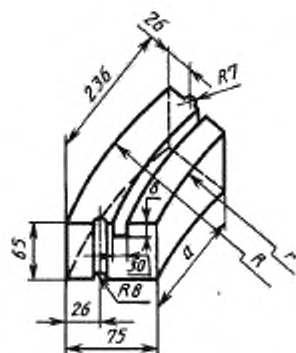
Рисунок 22 — Секторные изделия номеров 57—63
