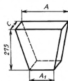
Рисунок 19 — Насадочные изделия номеров 43 — 48
