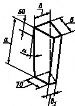
Рисунок 7 — Внешний электродный кирпич
