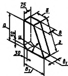
Рисунок 8 — Опорный кирпич
