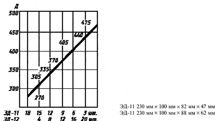
Рисунок В.1 — Свод толщиной 230 мм
