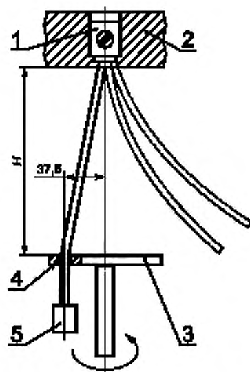
Рисунок 3 — Устройство для испытания прочности изоляции проводов
