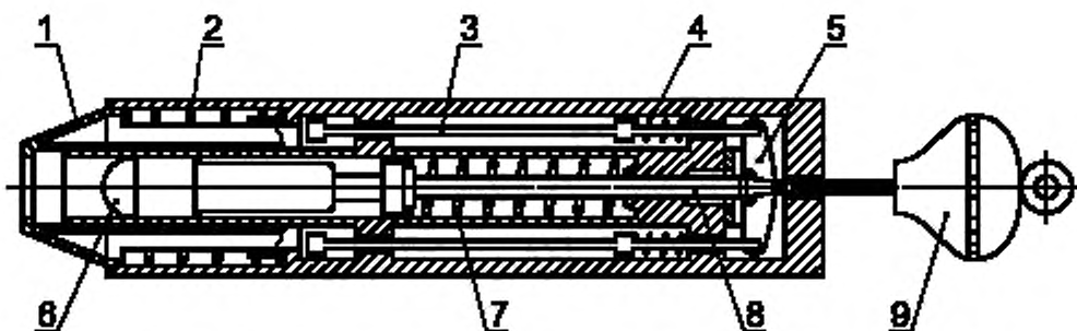
Рисунок 4 — Прибор для испытания на удар
