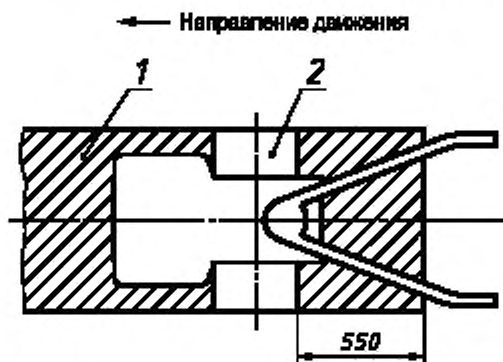
Рисунок 6 — Пределы опасной зоны в случае, когда устройство для запуска культиватора без реверсивной передачи
