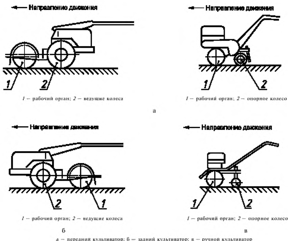
Рисунок 1 — Типы культиваторов
