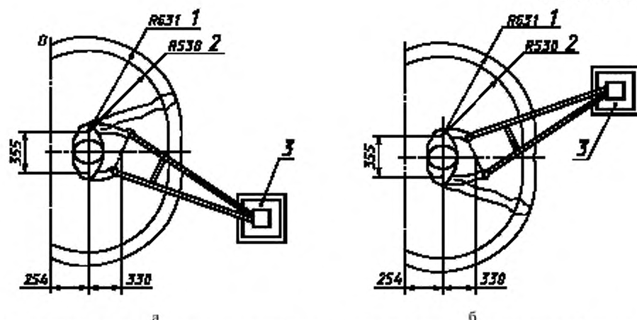
Рисунок 5 — Зона оператора, идущего рядом с культиватором
