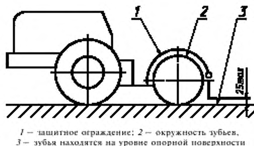
Рисунок 2 — Защита рабочего органа заднего культиватора
