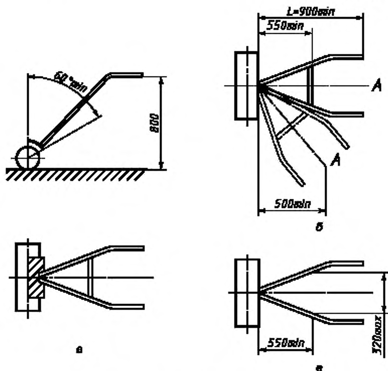
а — защитное ограждение (см. таблицу 1); б — рукоятки руля с поперечиной; в — рукоятки руля без поперечиной
