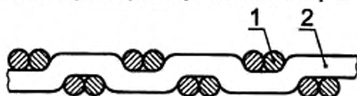
1 — нить основы ворсованная, 2 — нить утка ворсованная
