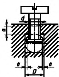
Зажим с прижимной пластиной
