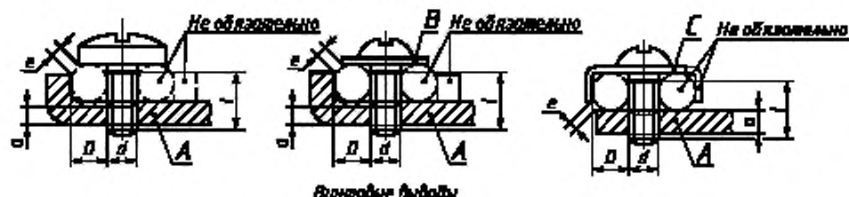
Винтовые выводы
