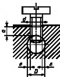
Зажим без прижимной пластины
