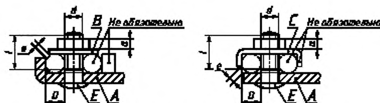
Болтовые выводы
