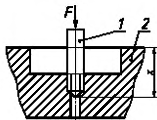
1 — штыревой калибр; 2 — головная часть штепсельной или переносной розетки
