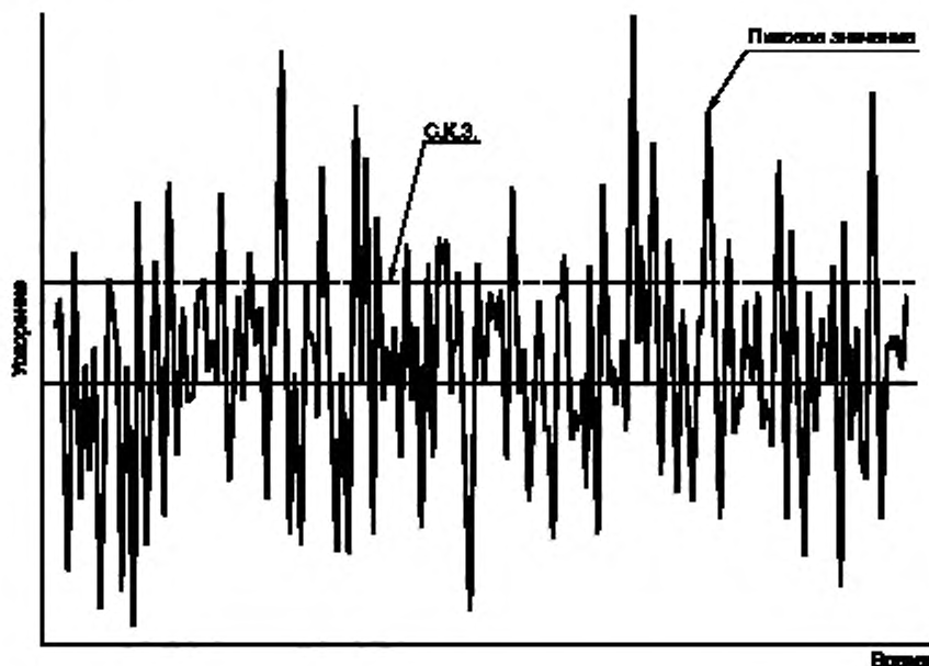
Рисунок А.2 — Отсечка (ограничение) сигнала
