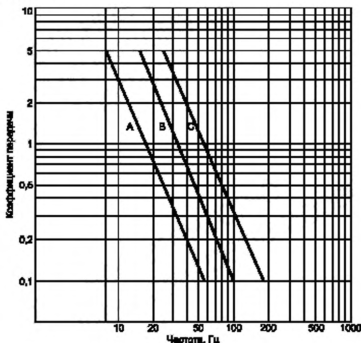
Рисунок A.6 — Коэффициент передачи виброизолятора
