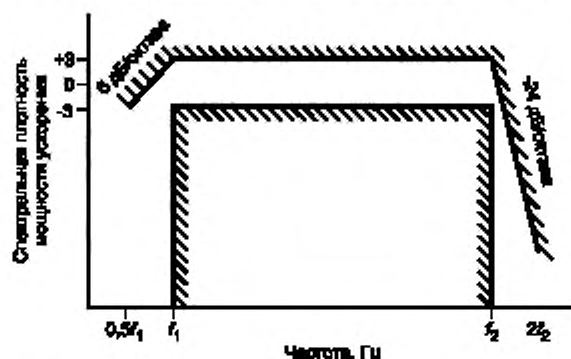
Рисунок 2 — Границы допуска для спектральной плотности мощности ускорения
