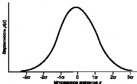
Рисунок А.1 — Гауссовская плотность распределения вероятностей
