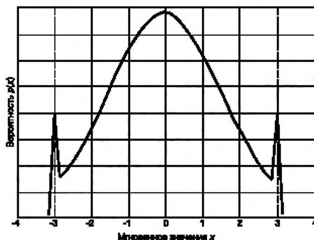
Рисунок А.3 — Негассовская плотность вероятности распределения
