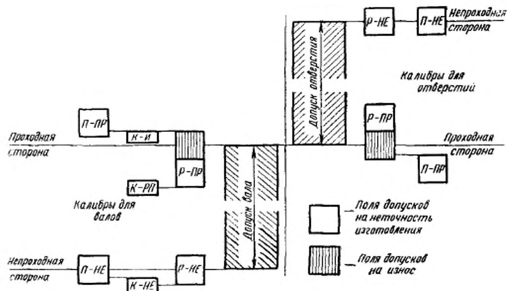
Схема расположения полей допусков калибров и контркалибров
