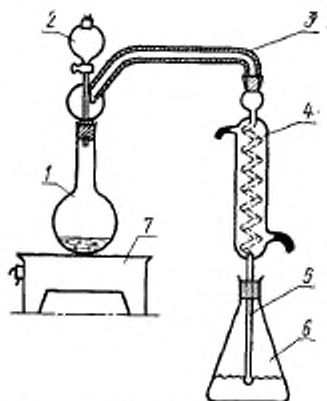
1—дистилляционная колба вместимостью 100 мл; 2—насадка с капельной воронкой; 3—дефлегматор с соединительной трубкой; 4—амперный холодильник; 5—барботер; 6—пробирка-приемник; 7—электроподставка.
