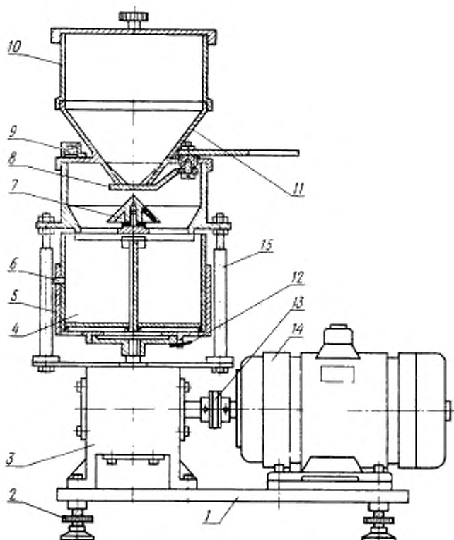
1—плата; 2—регулирующие винты; 3—червячный редуктор; 4—сектор; 5—обойма; 6—фиксатор; 7—усреднительный конус; 8—клапан; 9—уровень; 10—бункер; 11—дополнительный конус; 12—пружина; 13—муфта; 14—электродвигатель; 15—установочные стойки.
