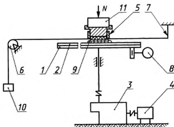
1 — опорный подвижный диск; 2 — образец; 3 — редуктор; 4 — приводной электродвигатель; 5 — цилиндрический короб; 6 — блок тарировочного устройства; 7 — тензобалка; 8 — тахометр; 9 — испытательная волокнистая масса; 10 — груз; 11 — тарировочный груз
