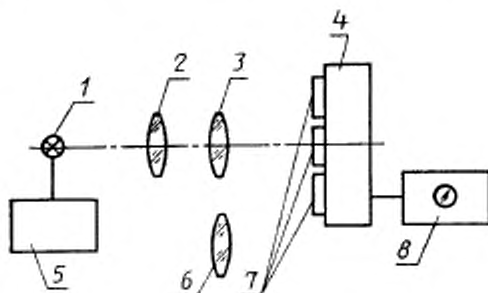
1 — источник света; 2 — коллиimator; 3 — эталонная насадка; 4 — фотоэлектрический колориметр; 5 — стабилизатор напряжения; 6 — испытуемая насадка; 7 — смешные светофильтры; 8 — измерительный прибор
