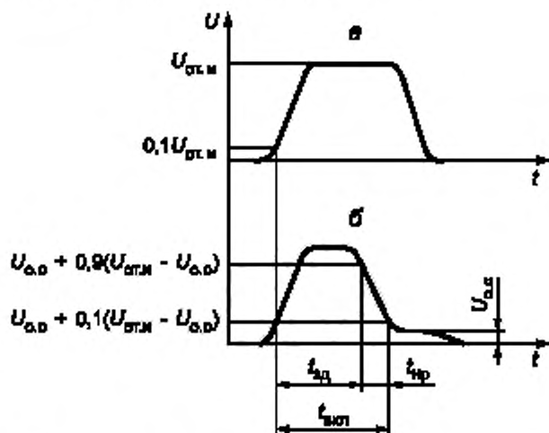
a — форма напряжения на выходе генератора GI при отсутствии испытуемого тиристора; b — форма напряжения на испытуемом тиристоре; U_{о.с} — постоянное напряжение в открытом состоянии тиристора; U_{отн} — импульсное отпирающее напряжение тиристора
