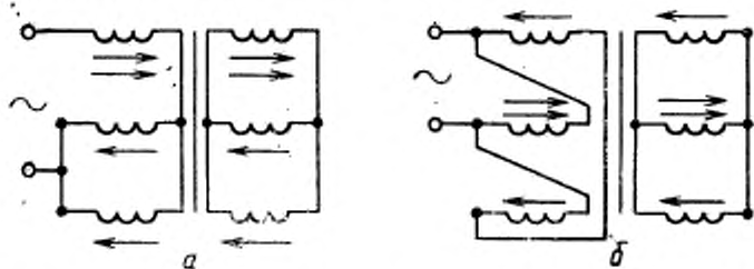
Две стрелки обозначена испытываемая фаза, по которой протекает ток КЗ вдвое больший, чем в двух других фазах.
