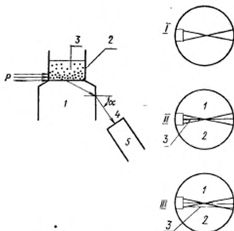
1 —призма; 2 —цилиндрическая линза, приклеенная к призме; 3 —смесь двух иммерсионных жидкостей с частями испытуемого материала; P —входящий луч света; 4 —выходящий из призмы луч света; 5 —зрительная труба рефрактометра; \alpha —предельный угол полного внутреннего отражения. I , II —поле зрения при совпадении и небольшом превышении показателей преломления испытуемого материала и иммерсионной жидкости соответственно; III —поле зрения при небольшом превышении показателя преломления иммерсионной жидкости над показателем преломления испытуемого материала; 1 —темная часть поля зрения; 2 —светлая часть поля зрения; 3 —граничная линия.
