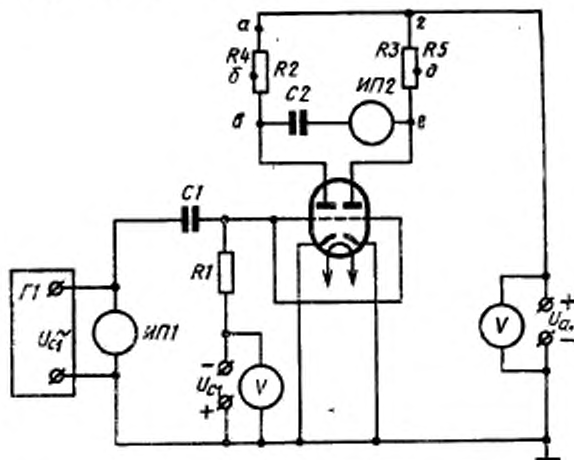
G1 — генератор синусоидального напряжения с частотой, фиксируемой в пределах от 400 до 1500 Гц; R1 — резистор; R2, R3 — безындукционные резисторы; ИП1 — вольтметр или делитель напряжения и вольтметр; ИП2 — вольтметр; C1, C2 — конденсаторы.
