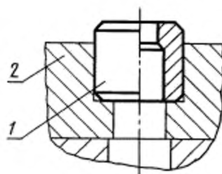
1 — матрица; 2 — державка
