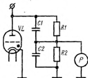
R_1, R_2 —резисторы; C_1, C_2 —конденсаторы; P —осциллограф; V_L —испытываемый тиристор.
