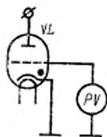
PV —измеритель напряжения, VI —испытываемый тиристор
