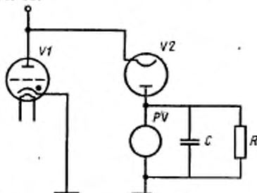
R —резистор; C —конденсатор; PV —измеритель напряжения; VI —испытываемый тиристор; V2 —диод
