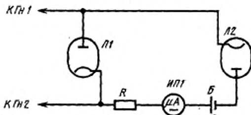
Принципиальная электрическая схема устройств измерения обратного тока
