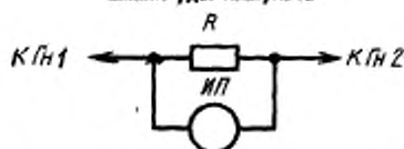
Принципиальная электрическая схема устройства измерения амплитуды импульса
