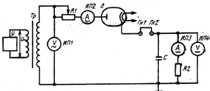
Принципиальная электрическая схема испытания одноанодных выпрямительных ламп на вентильную прочность
